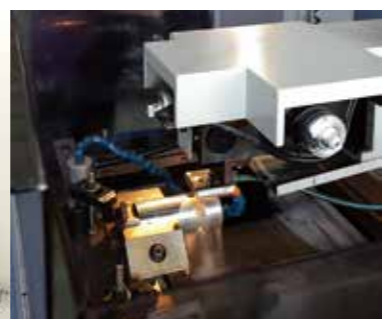
▲ 線切割機
